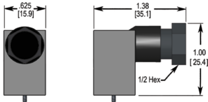
POS DIN CONNECTOR P/N 2270-0
