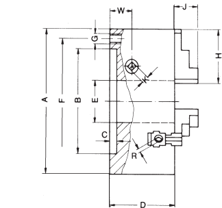
Cylindrical centre mount DIN 6351
