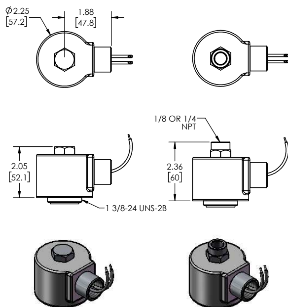
CONDUIT HOUSING
