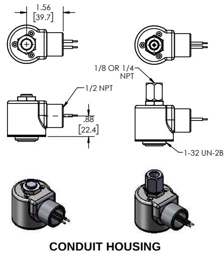
CONDUIT HOUSING
