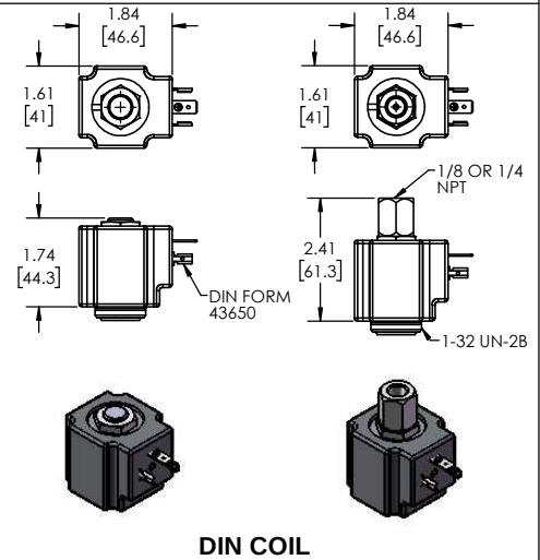
DIN COIL
