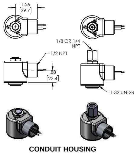
CONDUIT HOUSING
