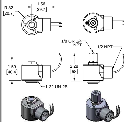
CONDUIT HOUSING
