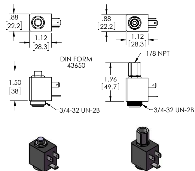
DIN COIL
